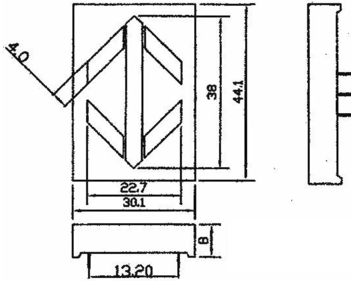
PCB-A
